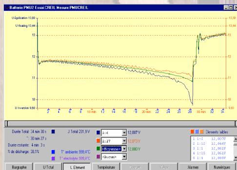
Courbes de décharge (tension totale ou tension des éléments)
